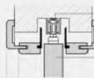
Holzschiebetür im Sturz
