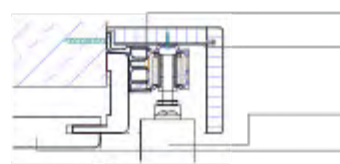
Montage mit Schiebetürfutter für Holztür
