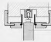
Holzschiebetür im Sturz
