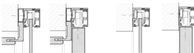
Montage ohne DUFU
