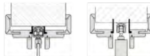
Deckenmontage unter Sturz
