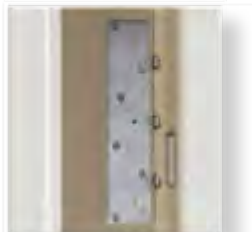
verstärktes Schließblech mit Stahlhalterplatte Nr. 35 Ansicht Futterrückseite
