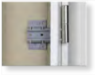
2-teiliges Bandsystem V3420 WF Tragfähigkeit einer Standard-Türe bis 40 kg
